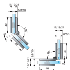
8775 verstellbarer Winkelverbinder Glas-Glas 135°
