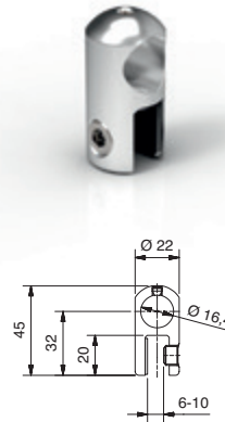
für Rohr Ø 16 mm
