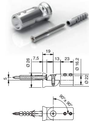
für Rohr Ø 16 mm
