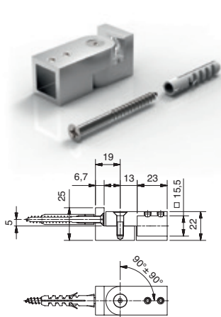
für Rohr □ 15 mm
