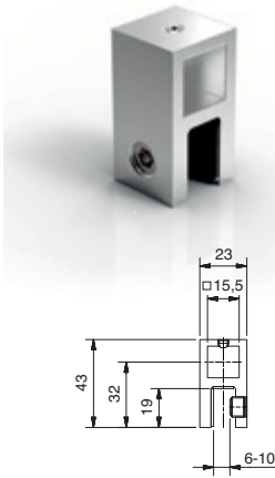
für Rohr □ 15 mm
